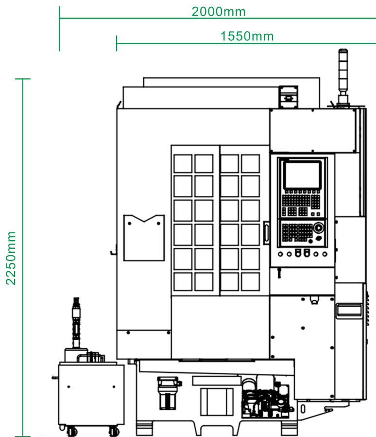
前视图
