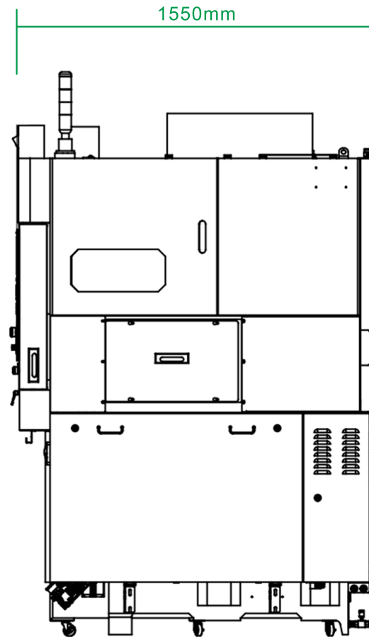
侧视图
